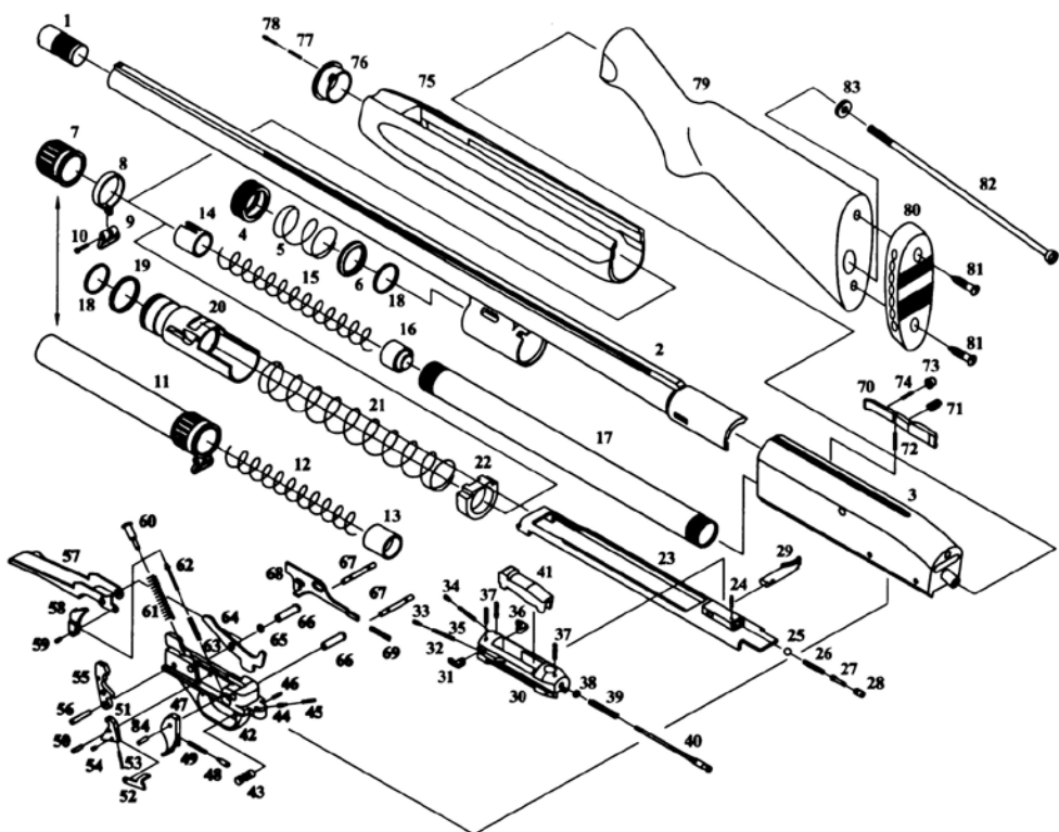
Рисунок 2 – Сборочные единицы и детали ружья
